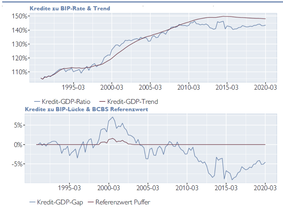
Grafik 1: Verlauf Kredit/BIP-Lücke
