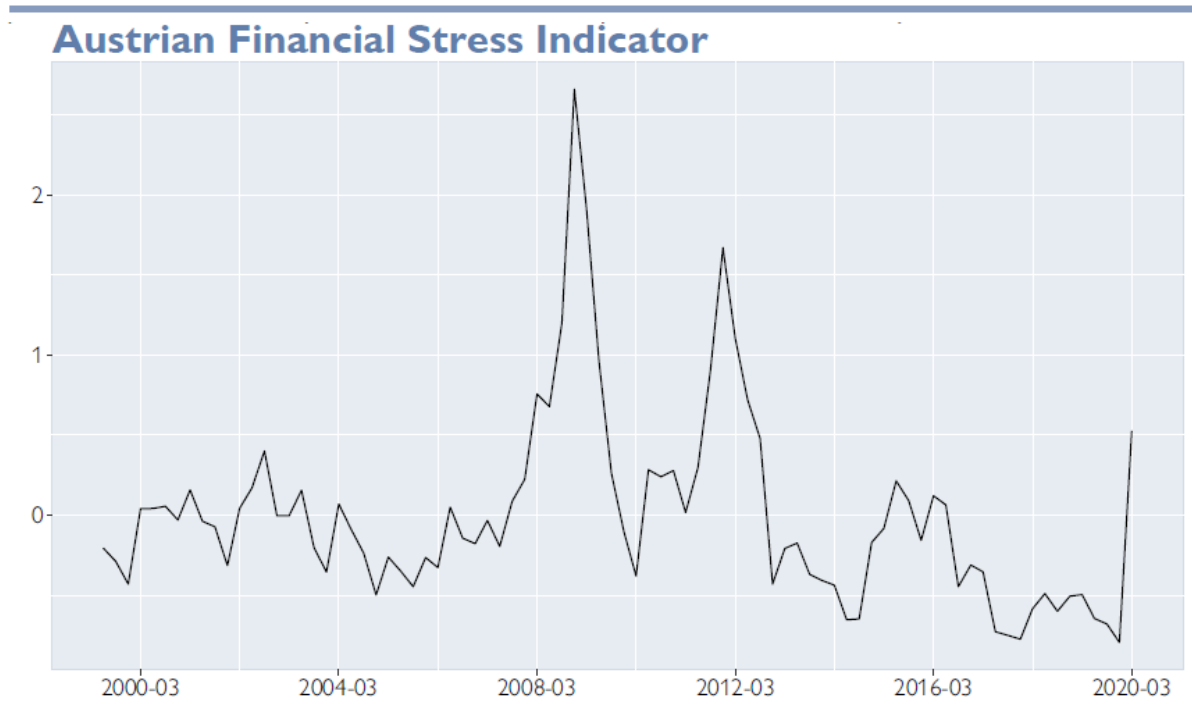
Grafik 2: Verlauf Austrian Financial Stress Indicator
